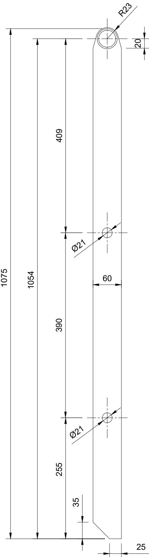
Detail pos. 6
