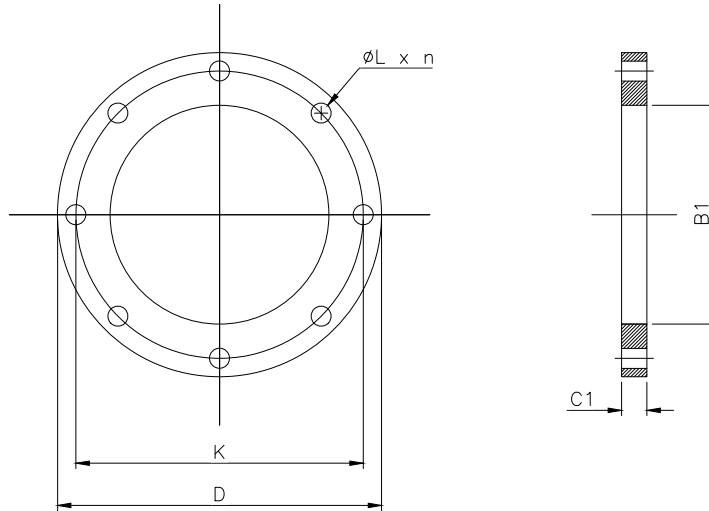
DIMENSIONS OF PN 40 FLANGES
