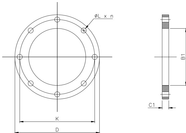
DIMENSIONS OF PN 25 FLANGES
