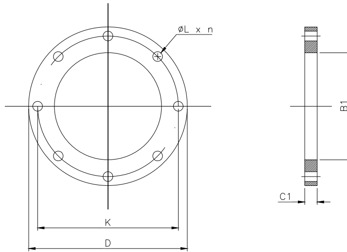
DIMENSIONS OF PN 16 FLANGES
