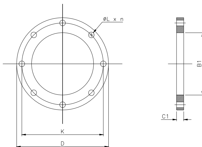
DIMENSIONS OF PN 6 FLANGES
