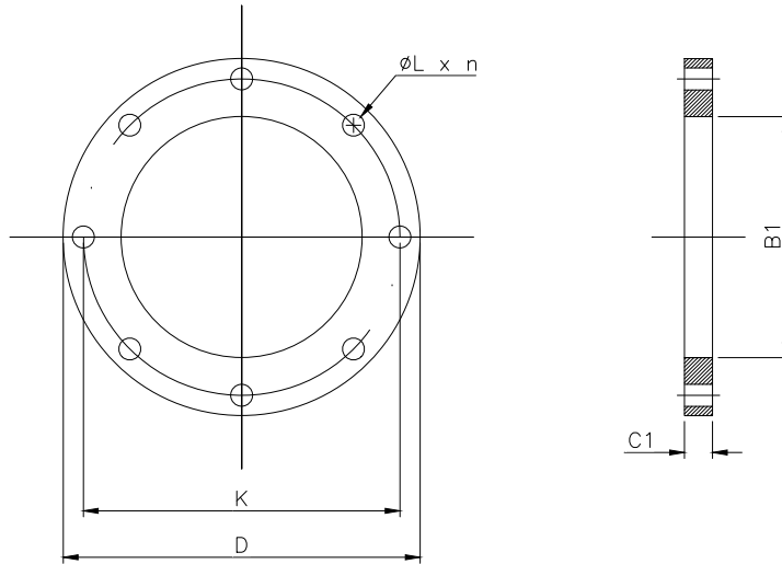
DIMENSIONS OF PN 10 FLANGES
