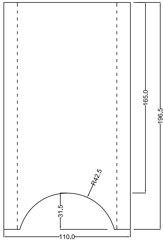
ELEVATION
